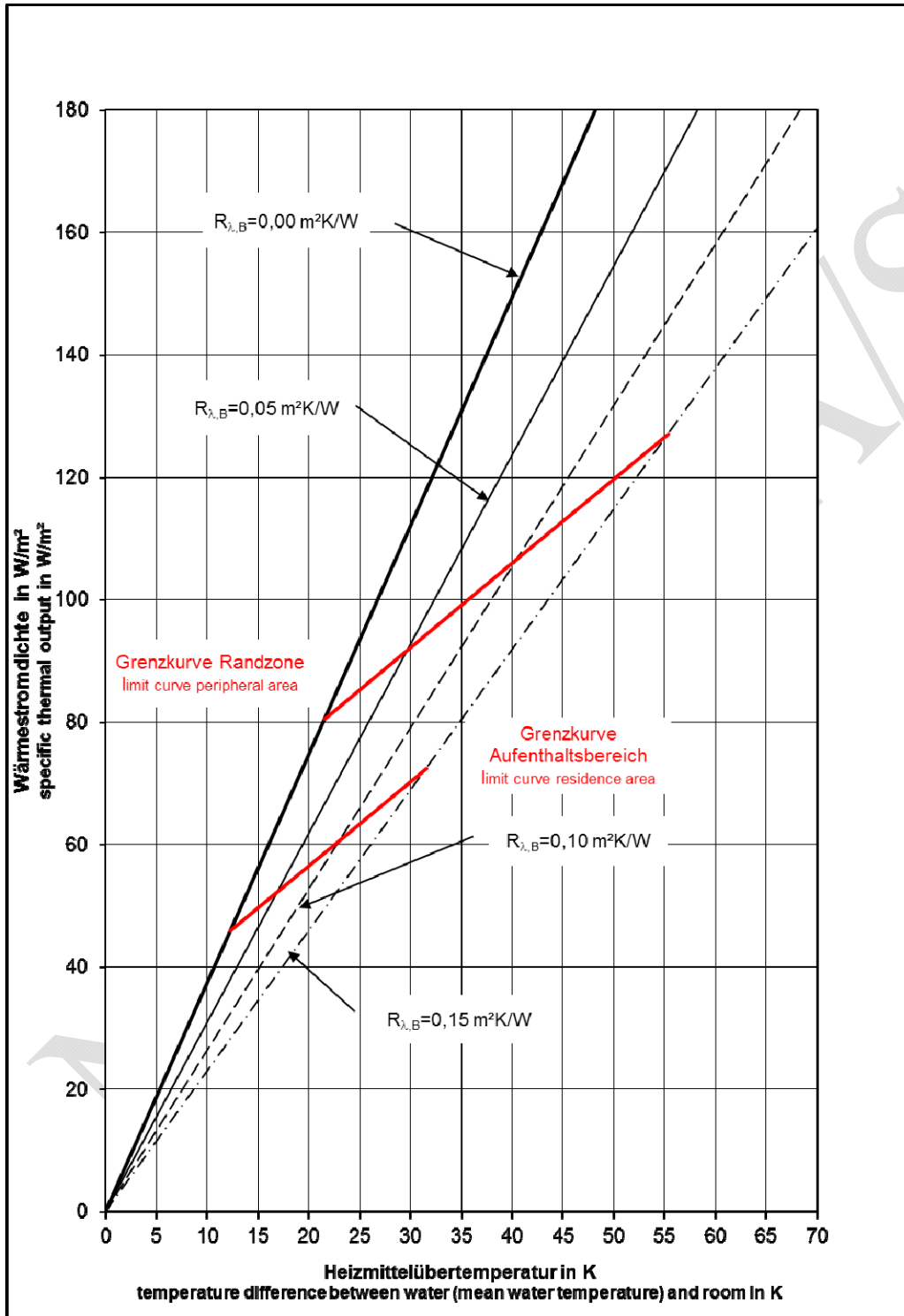
Abbildung 5: Leistungskennlinien Fußbodenheizungssystem
